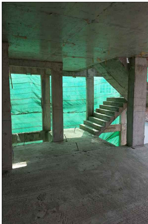
ระบบพื้น POST-TENSION และ โครงสร้างบันได
